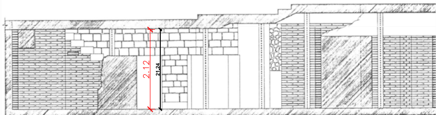
Secció A-A'
