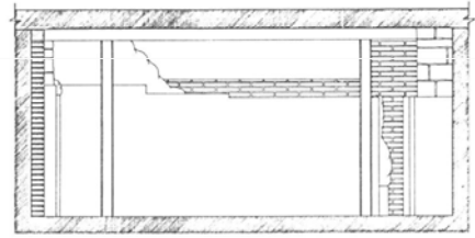
Secció B-B'
